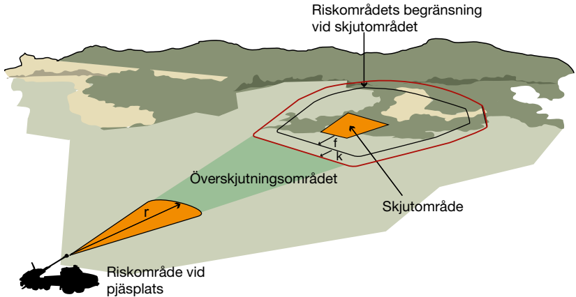
Bild 4.2. Exempel på delat riskområde
