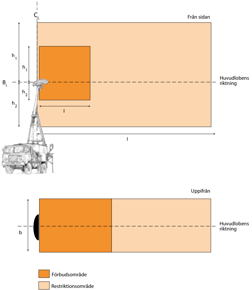
Bild 7.2. Måttsättning vid bestämning av förbuds- eller restriktionsområde vid stillastående eller sakta svepande antenn
