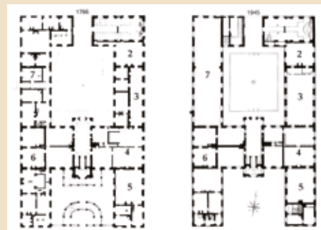
Rumsindelning 1766 och 1945
